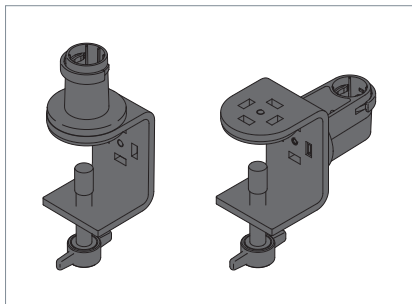
Fig. 3: Pincettes de table.
